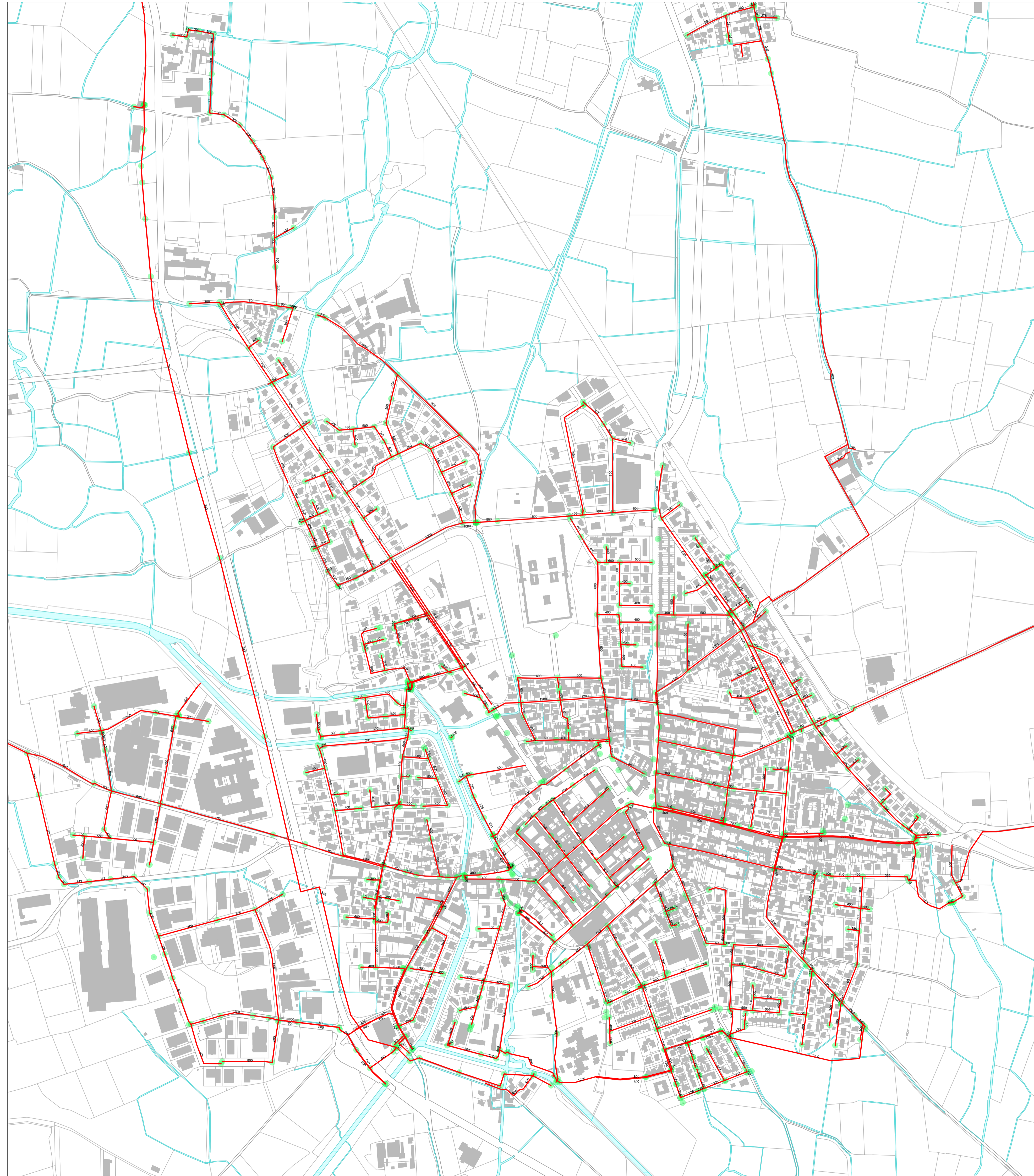
Sviluppo sistema fognario - Capoluogo SCALA 1:5000
